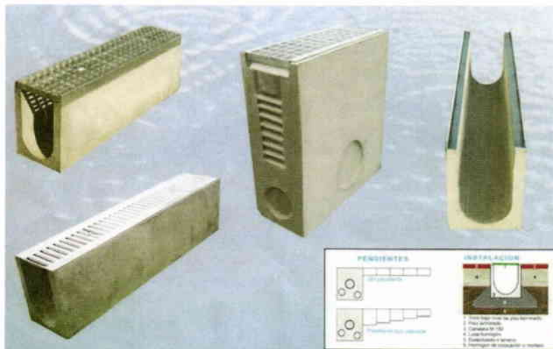
Figura 3: Canaletas recolectoras de aguas lluvias.
